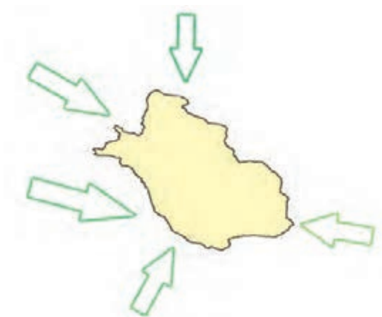
شکل ۱۷-۱- نقشه مسیر ورود توده‌های هوا به استان
