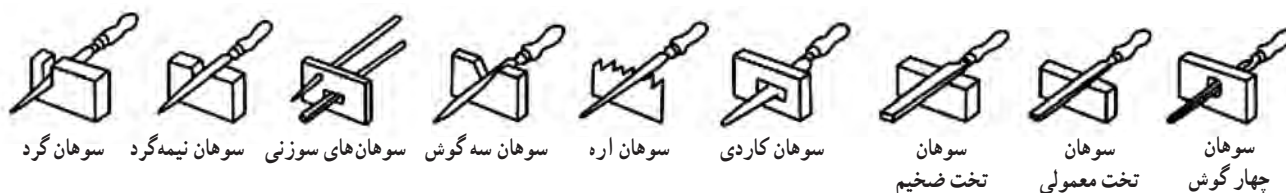
شکل ۵-۱۴. انواع سوهان در شکل‌های متفاوت
