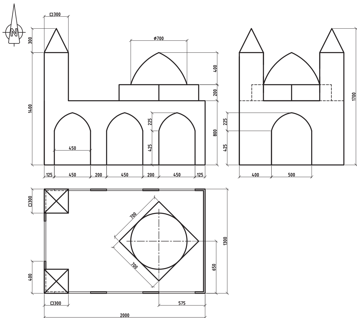
شکل ۱۲-۹. نقشه نمای مسجد
