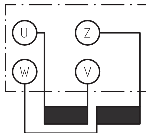
شکل ۲۱- استاندارد VDE
