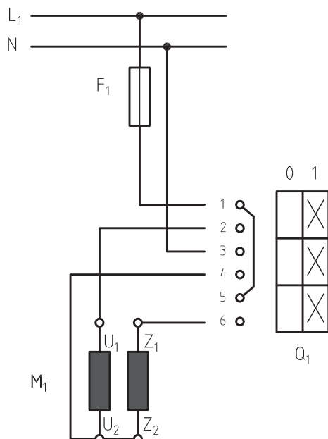
شکل ۲۳- راه اندازی موتور تک فاز با کلید زبانهای
