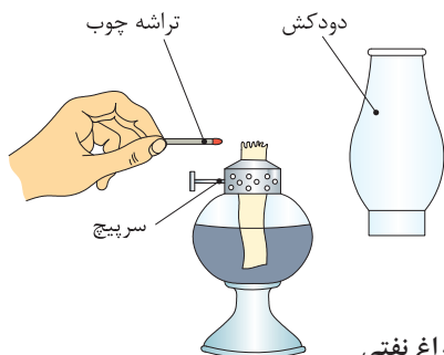
شکل ۳۲- چراغ نفتی
