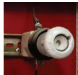
شکل ۱۴- فیوز فشنگی
