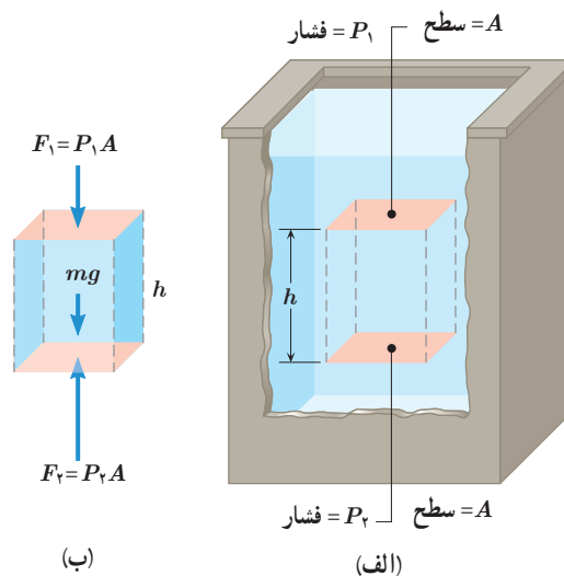
شکل ۲-۱۴ الف) بخشی از شماره ساکن (ب) نیروهای وارد بر این بخش از شماره در راستای قائم.
