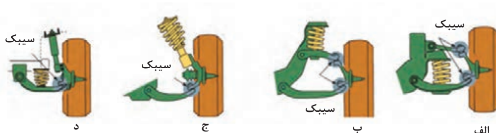
شکل ۱۳- انواع محل قرارگیری سبیک
