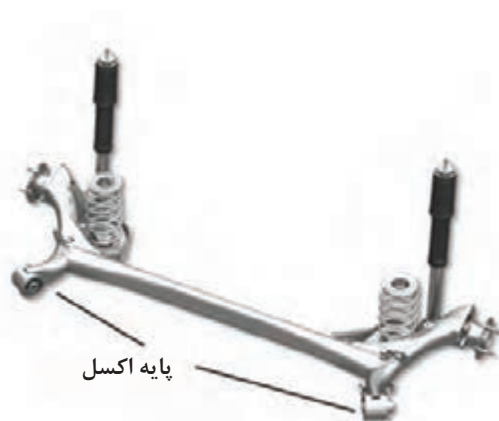
شکل ۴۴- نوعی تعلیق مرکب
