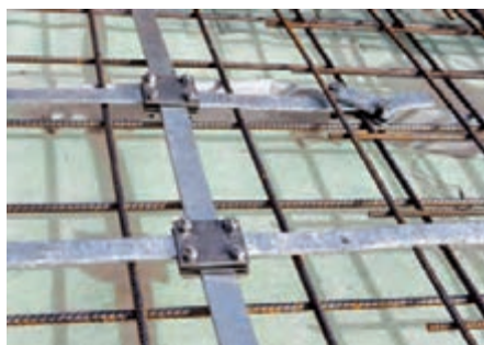
شکل ۹ – تسمه همبندی
