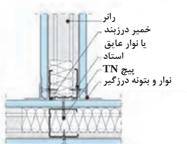
شکل ۷۴-۱. جزئیات پلان از اتصال دو دیوار یک لایه به یکدیگر (اتصال T)
