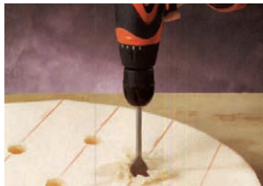
شکل ۴-۵۷- سوراخ‌کاری محل لmse
